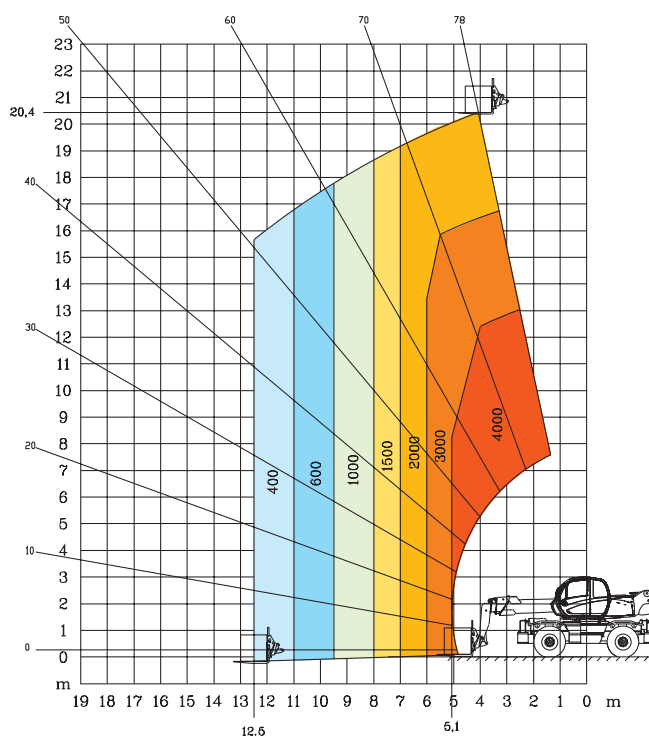
Frontale su pneumatici con forche
